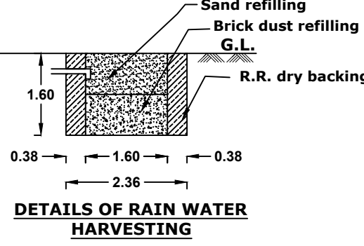
SOAK PIT
