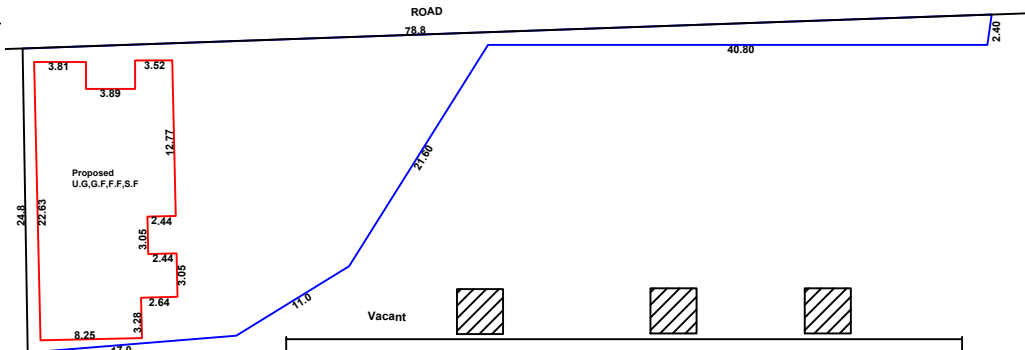
SITE PLAN 1:100
