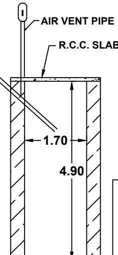
SOAK PIT
