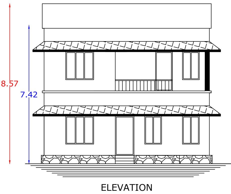
ELEVATION
