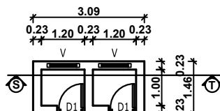
TOILET PLAN
