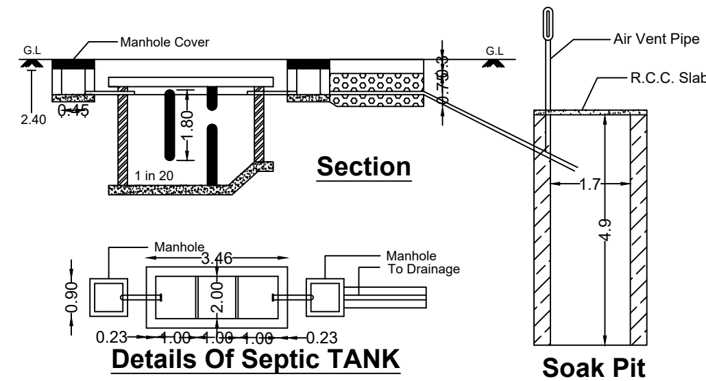
Soak Pit
