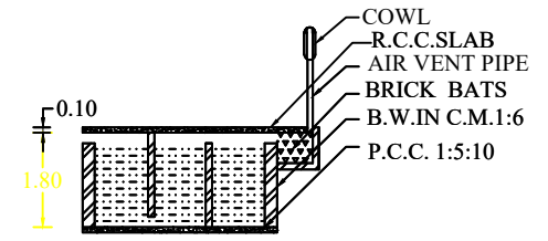
S.T. SECTION
