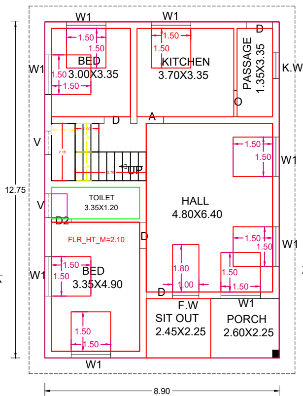
G.F.PLAN
