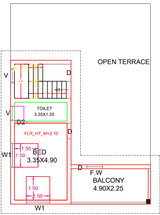
F.F.PLAN
