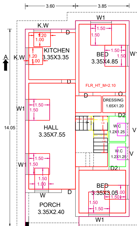
G.F.PLAN
