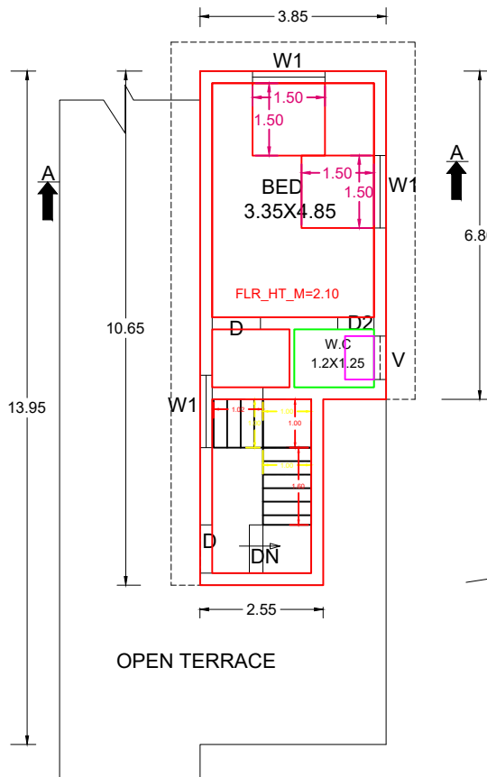
F.F.PLAN
