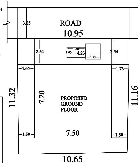
SITE PLAN 1:100
