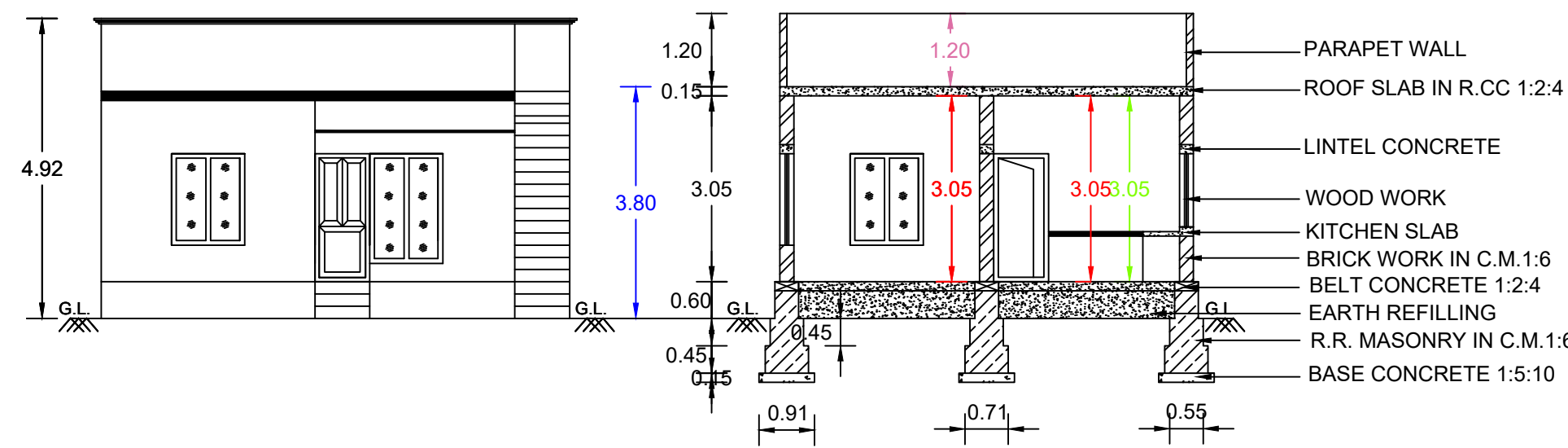
ELEVATION
