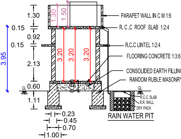
SECTION - AB
