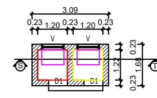
TOILET PLAN
