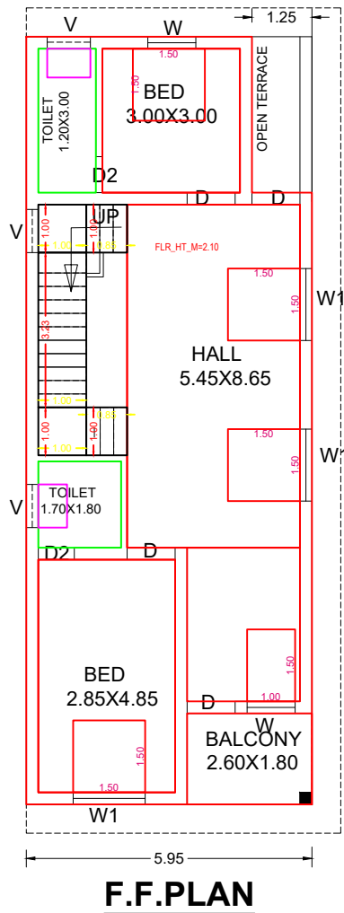
F.F.PLAN
