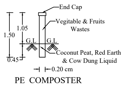
PE COMPOSTER
