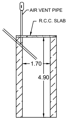
SOAK PIT
