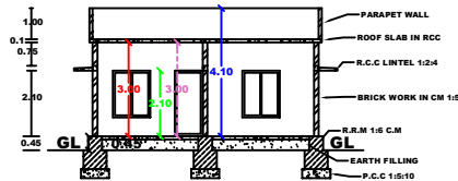
SECTION -AB
