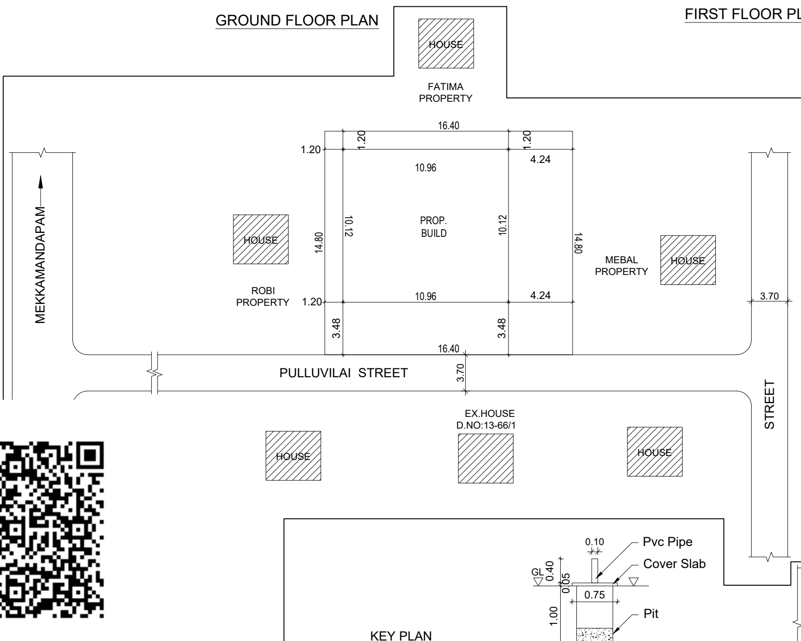
KEY PLAN SCALE:1:200.
