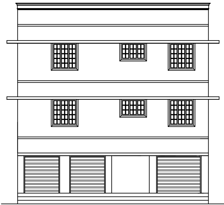
ELEVATION
