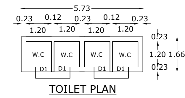
TOILET PLAN
