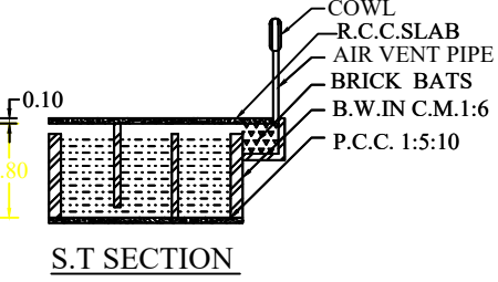
S.T SECTION
