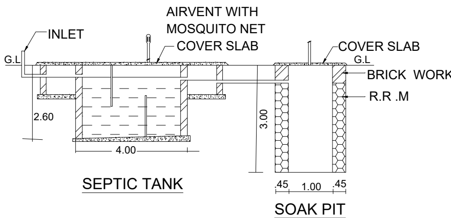
SOAK PIT
