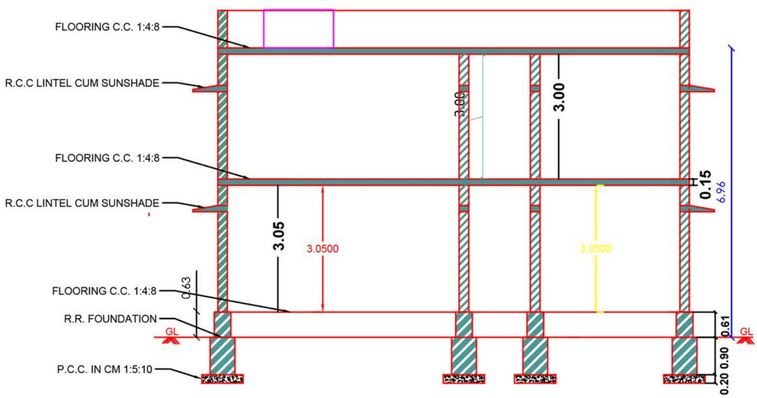
SECTIONN A-A
