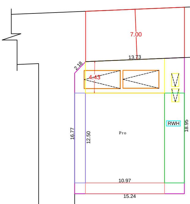
SCALE 1:100 SITE PLAN
