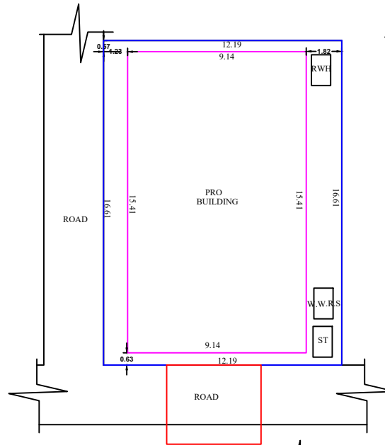
SITE PLAN 1:100
