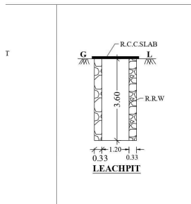
LEACH PIT R.C.C.SLAB R.R.W. 1.20 0.33 0.33
