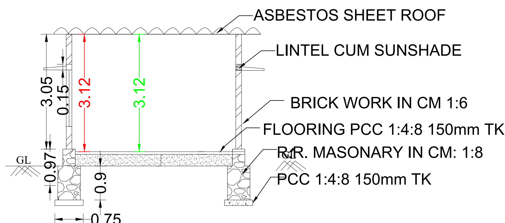
SECTION A-A
