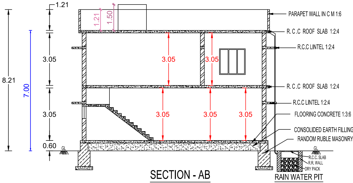
SECTION - AB
