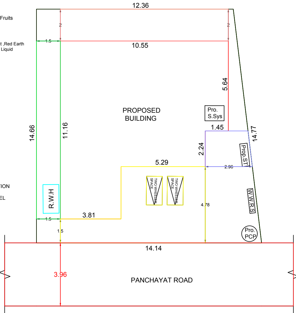
SITE PLAN 1:100
