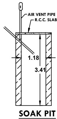
SOAK PIT
