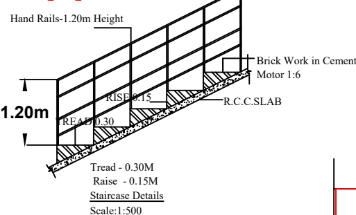
Staircase Details Scale: 1:500
