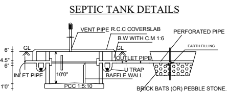
SECTION ON S.P.T & D.T
