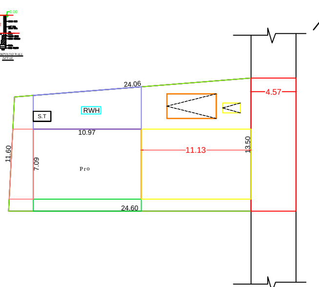
SCALE 1:100 SITE PLAN
