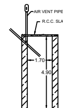
SOAK PIT
