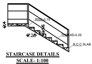
STAIRCASE DETAILS SCALE: 1:100
