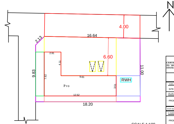
SCALE 1:100 SITE PLAN
