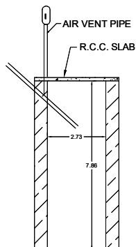
SOAK PIT
