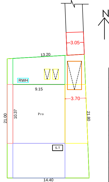
SCALE 1:100 SITE PLAN
