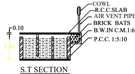
S.T. SECTION
