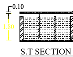
S.T. SECTION
