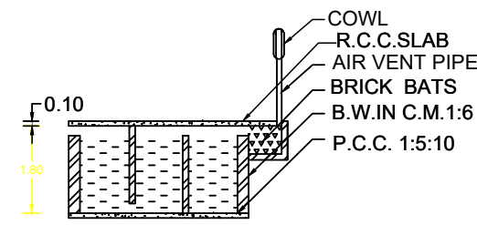
S.T SECTION
