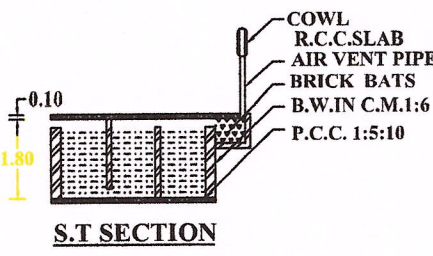
S.T. SECTION
