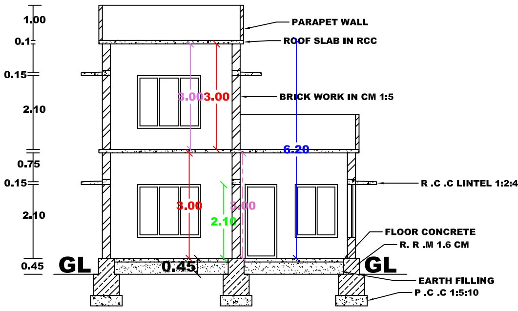
SECTION -AB
