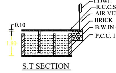
S.T SECTION
