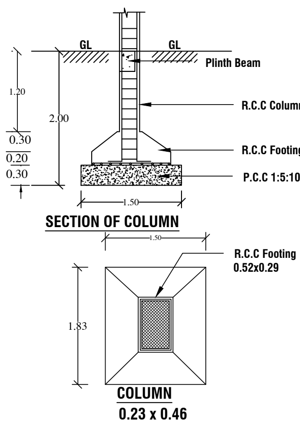
COLUMN 0.23 x 0.46
