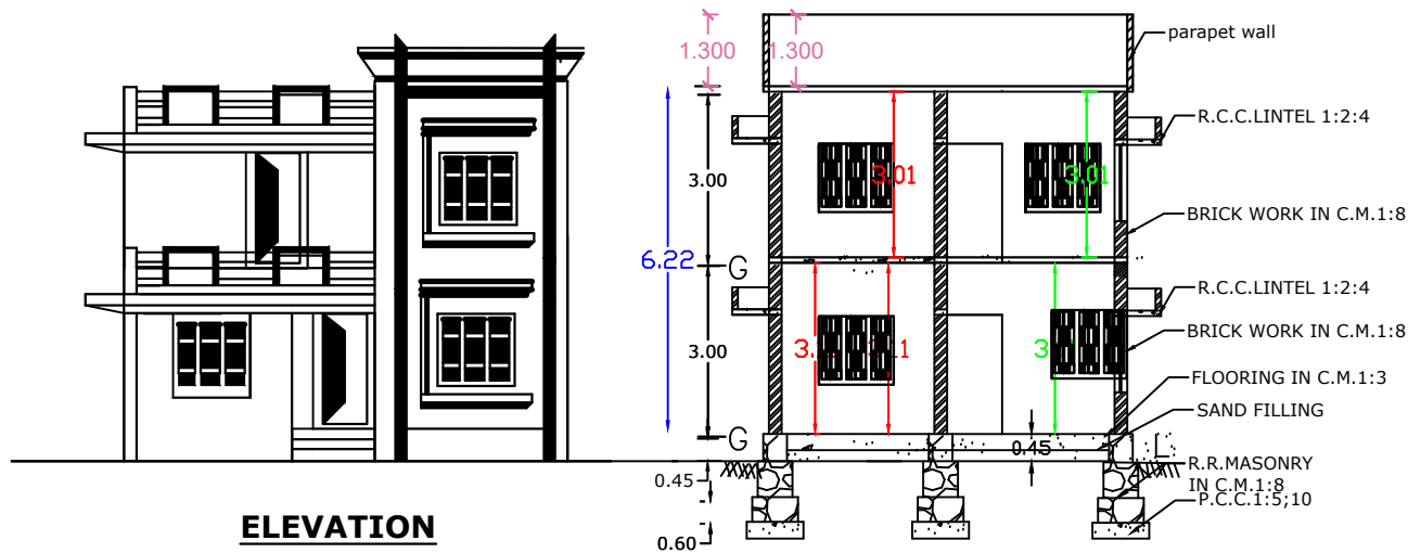
ELEVATION
