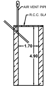
SOAK PIT
