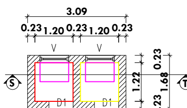
TOILET PLAN
