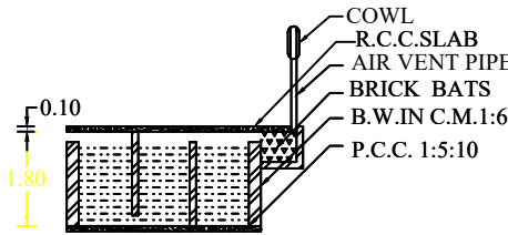
S.T SECTION
