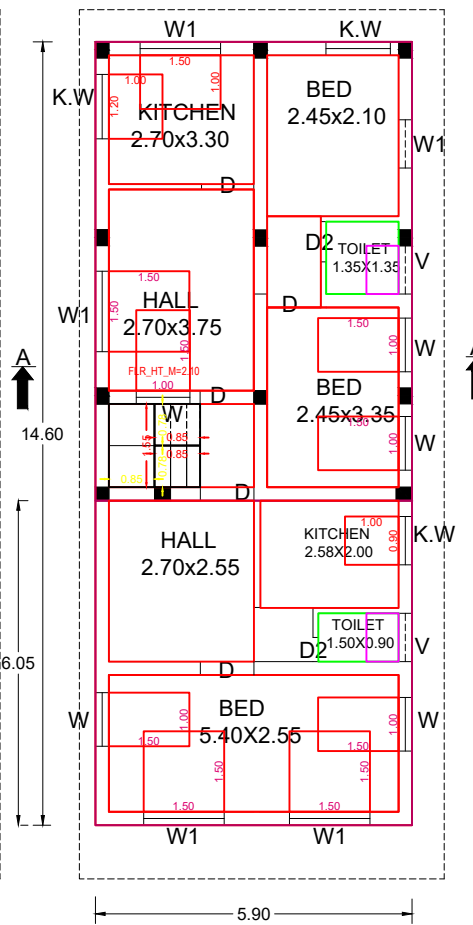
F.F. PLAN
