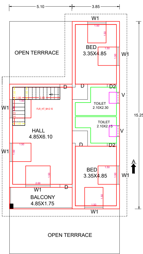
F.F.PLAN
