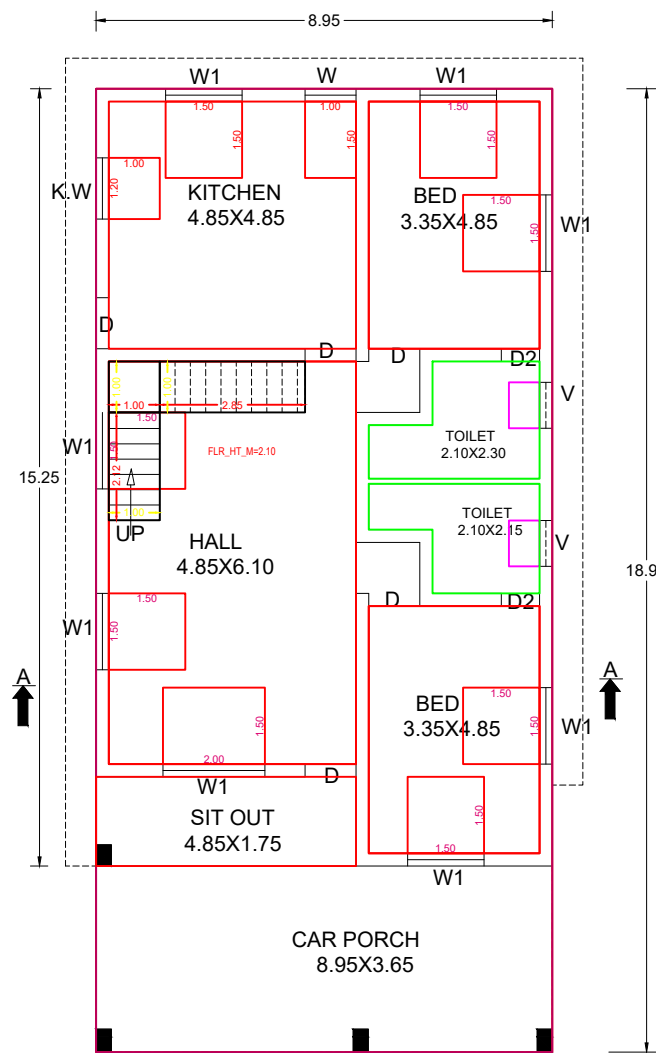
G.F.PLAN
